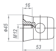
C3-53 Полуконнектор конусный Вес: 0,15 кг
