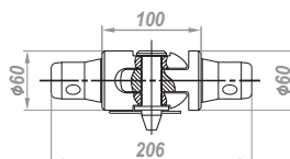
C3-100HV/HH Коннектор шарнирный Вес: 1,1 кг
