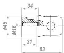
C3-83 Полуконнектор конусный Вес: 0,27 кг
