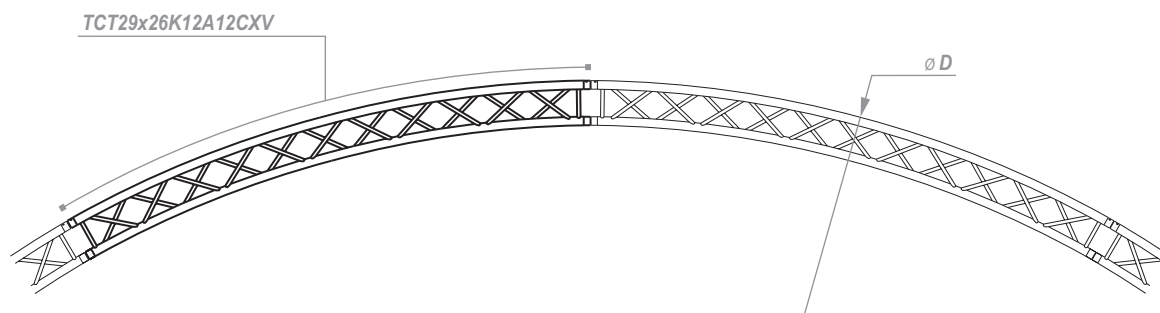
Рисунок 1 - фрагмент круга из треугольных ферм серии T29
